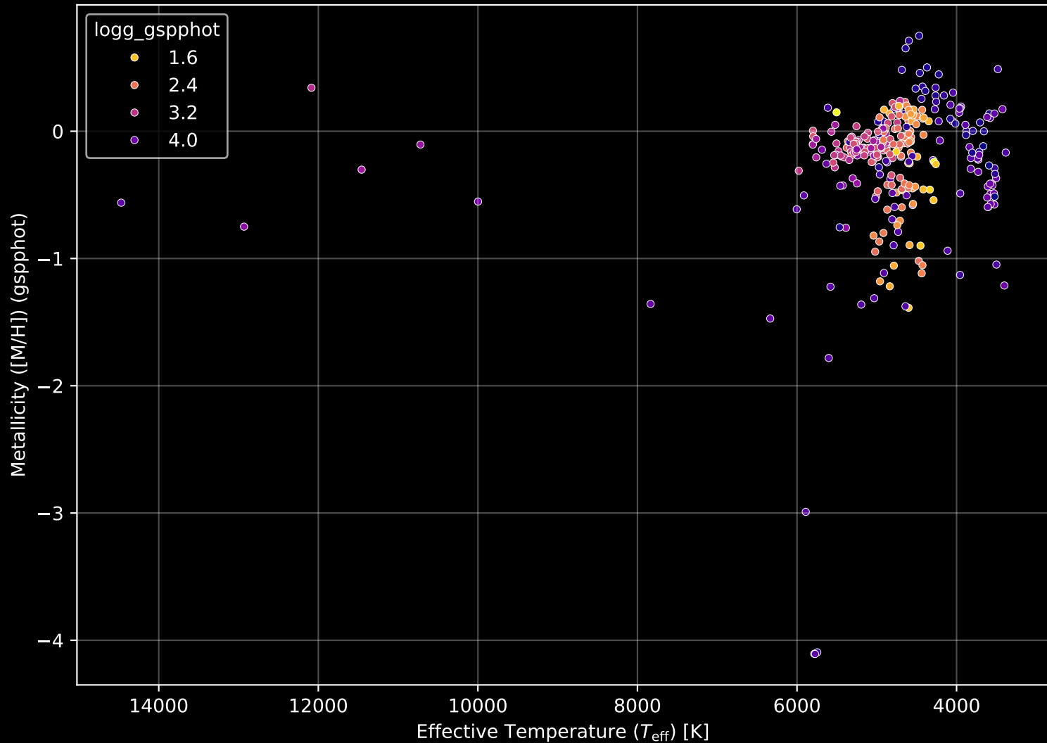
APOGEE DR17 Field: [Berkeley_20_btx] Stellar Population Parameters (n= 309)
